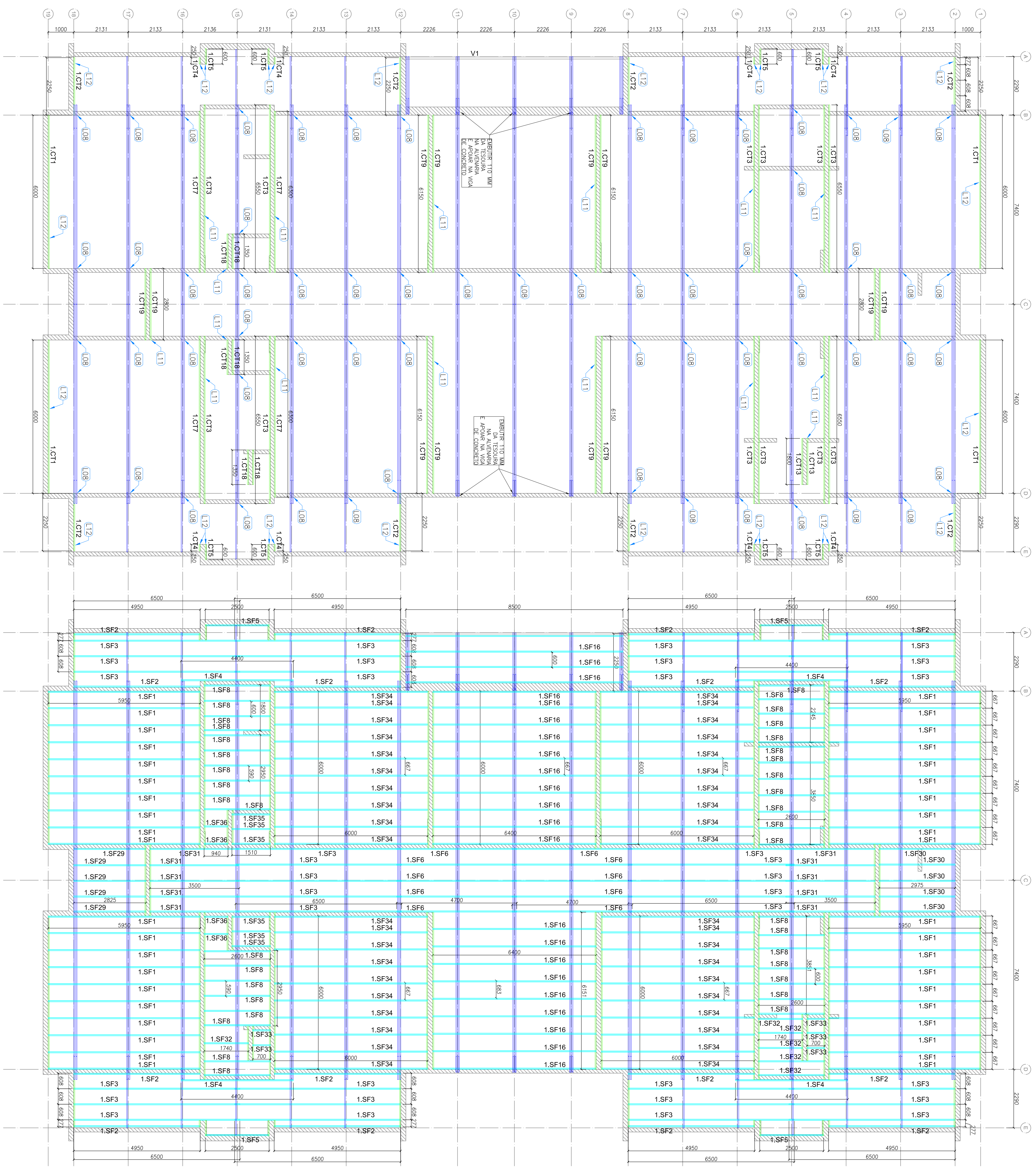
1 BLOCO B - VISTA EM PLANTA - CANTONEIRAS DO FORRO ESCALA: 1/75
