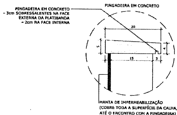
Figura 2-Detalhamento da pingadeira. Fonte -FNDE 2013
