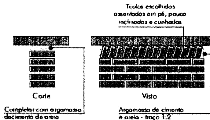
Figura 2 - Detalhamento de encunhamento. Fonte - FNDE 2013
